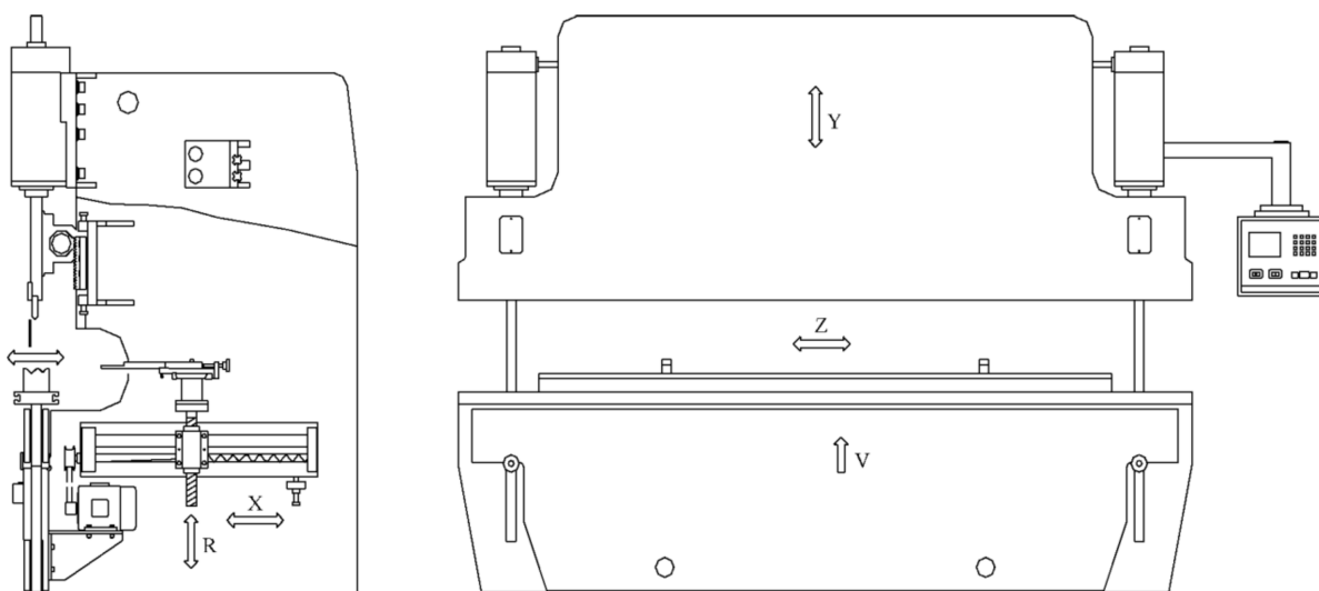
图 1 数控折弯机常用各数控轴示意图
